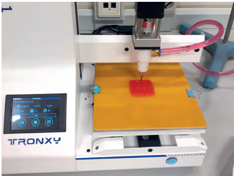
Equip d'impressió 3D per deposició adaptat a aliments
